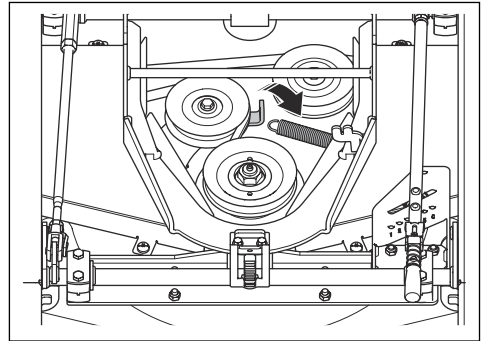
Aperçu de la courroie - R137, R137X
